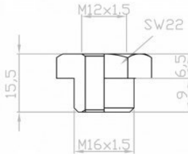
N092 M16/M12- AG/IG 053.16.12.105 Nippel zuignap, verloop, M16x1,5 AG, M12x1,5 IG
